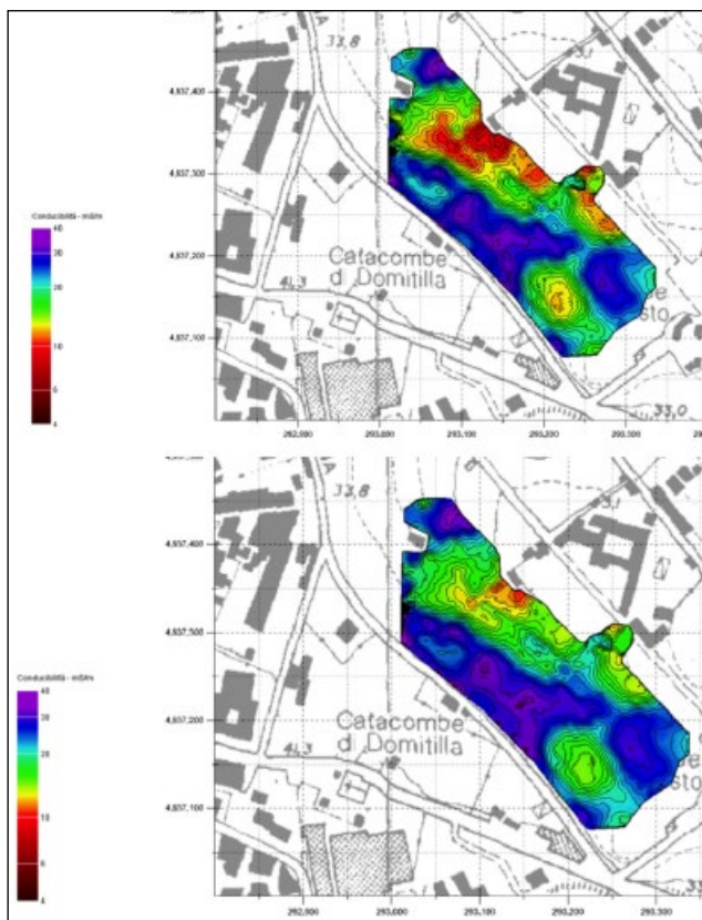
Fig. 15 – Mappe di conducibilità elettromagnetica.
