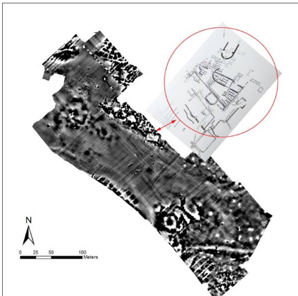
Fig. 5 – Magnetogramma con evidenziata l'area nella quale si rileva sovrapposizione con le strutture portate in luce dagli scavi novecenteschi dell'area sopratterra della cataomba di Marco e Marcelliano (SPERA 1999, 88).
